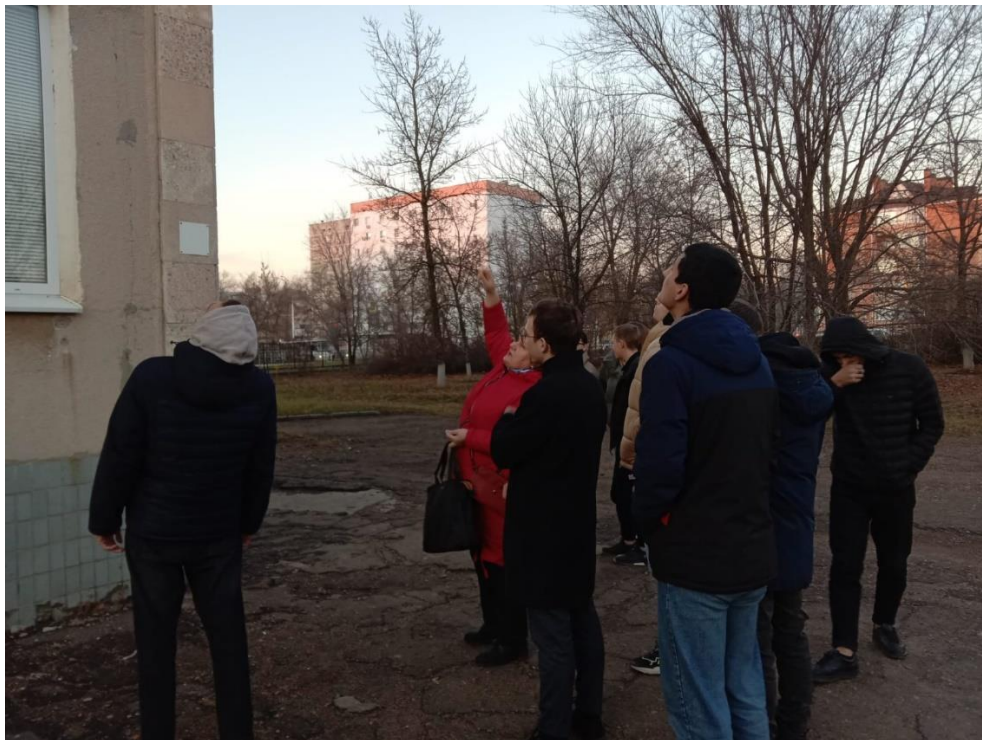
Рис. 4 Деформационные трещины на стыке стеновых панелей.
